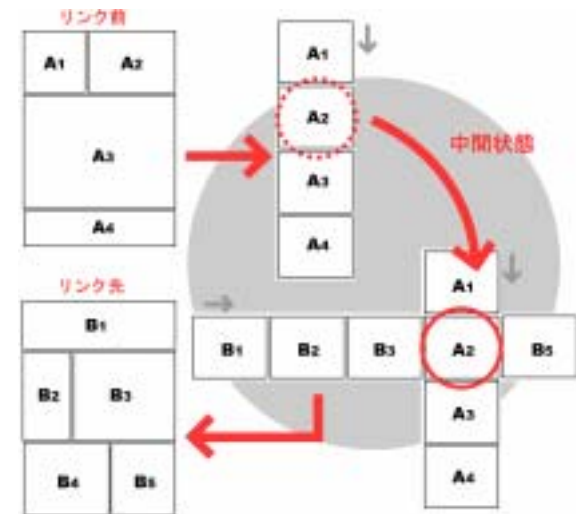
画面遷移図
